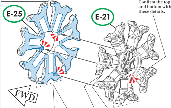
前列シリンダーブロック Front Cylinder Block
