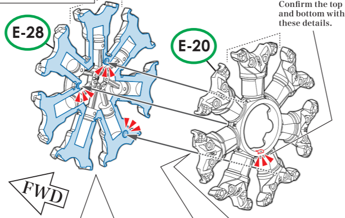
後列シリンダーブロック Rear Cylinder Block
