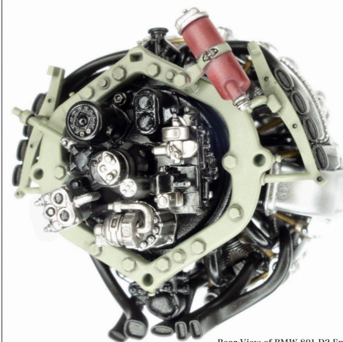
Rear View of BMW 801 D2 Engine / BMW 801 D2 エンジン 背面側
