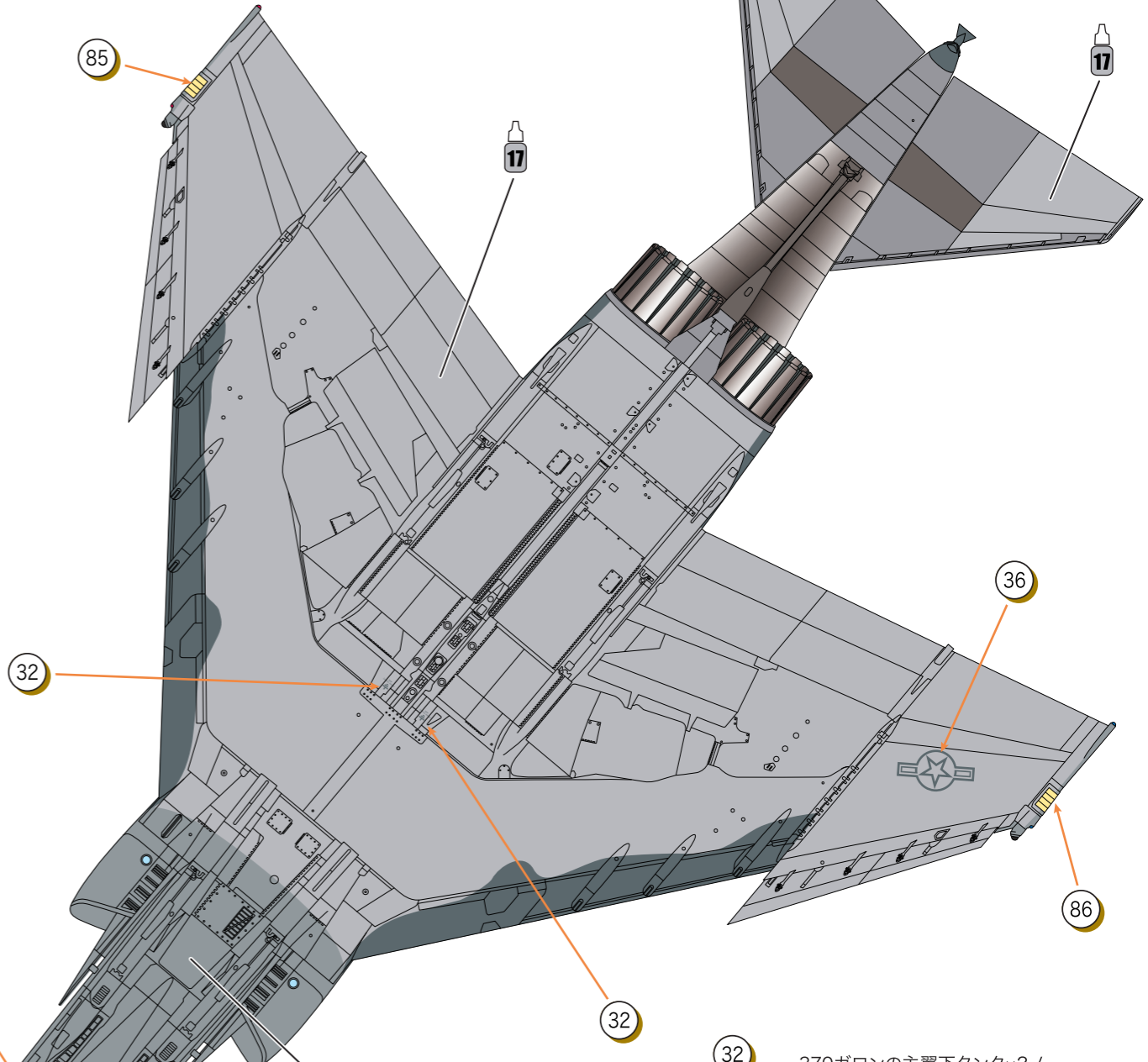
370ガロンの主翼下タンクx2 / 370 gal auxiliary wing tanks (2x)
