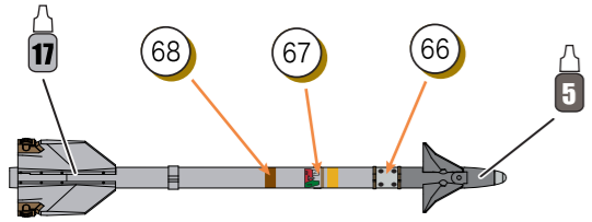
AIM-9L/M サイドワインダーミサイル x4 / AIM-9L/M Sidewinder missiles (4x)
